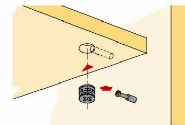
Рис.2 Схема сборки стяжки эксцентриковой
