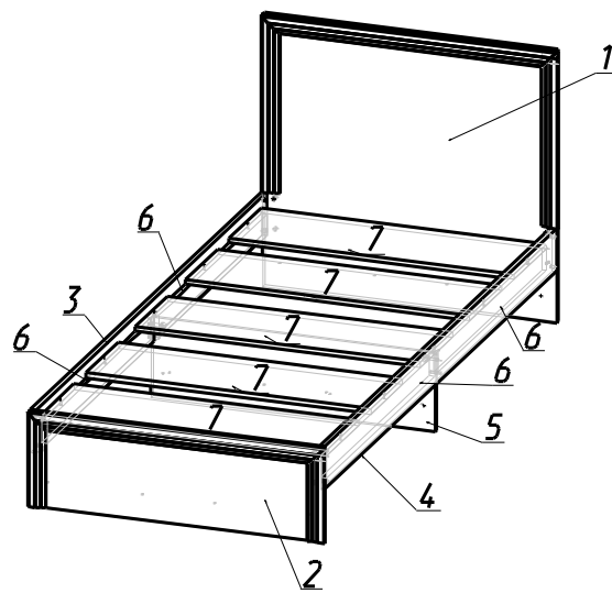
Рис.1 Схема сборки
